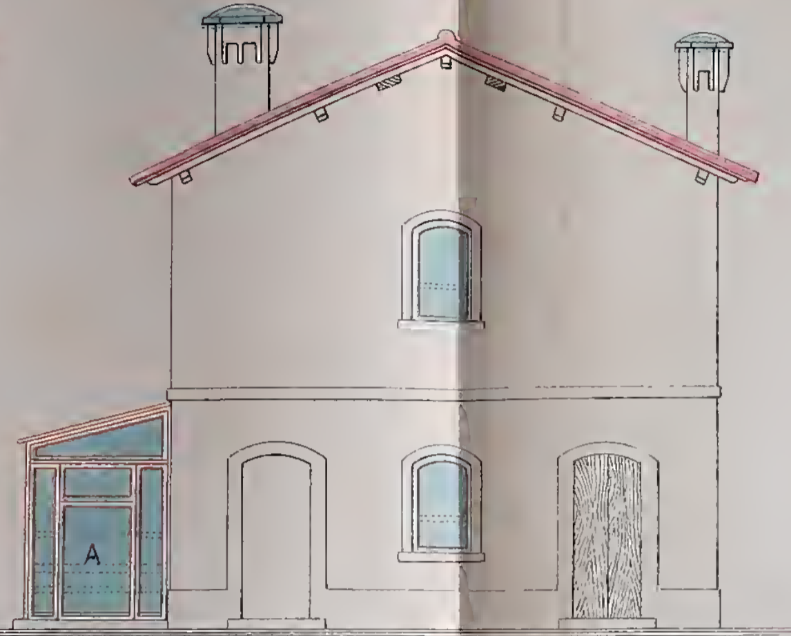
Fianco
